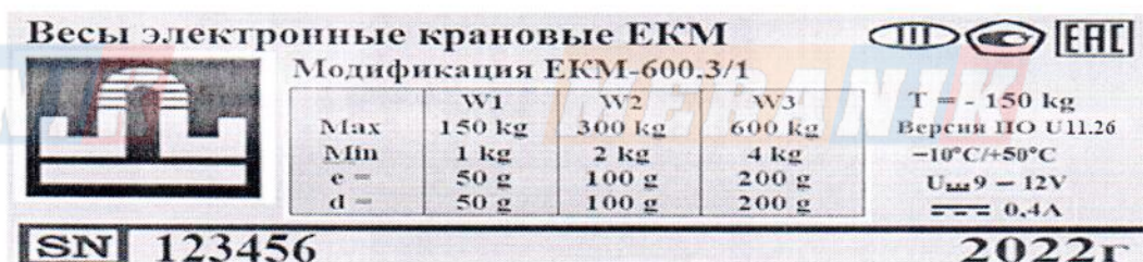
Рисунок 2 – Маркировка весов
